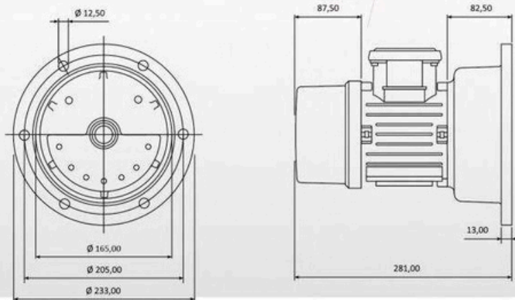
Gövde Ölçüleri - Overall Dimensions (mm)
