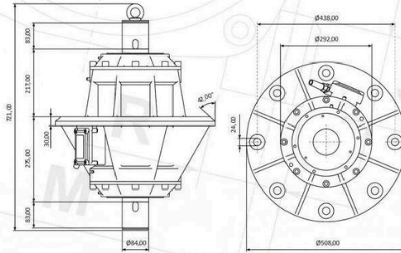
Gövde Ölçüleri - Overall Dimensions (mm)
